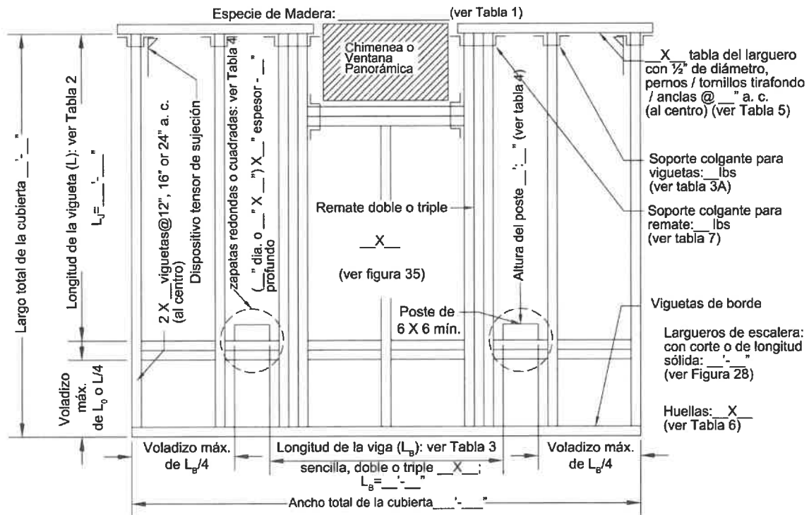
Figura 5. Plano Típico de Estructura de Cubierta.
