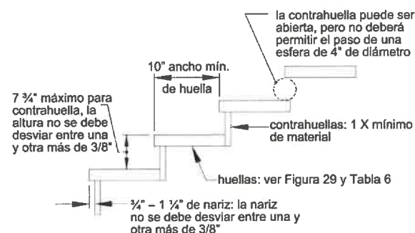
Figura 27. Detalle de Huella y Contrahuella.
