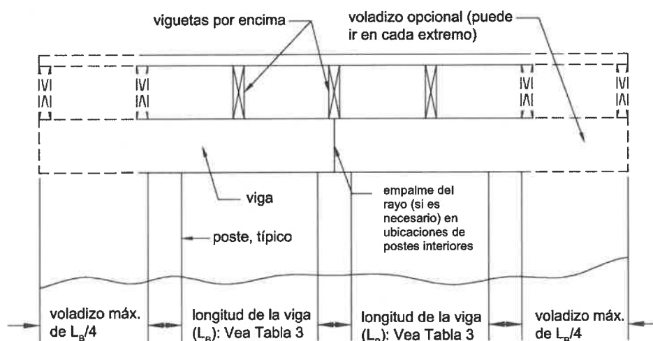
Figura 3. Longitudes de Vigas.
