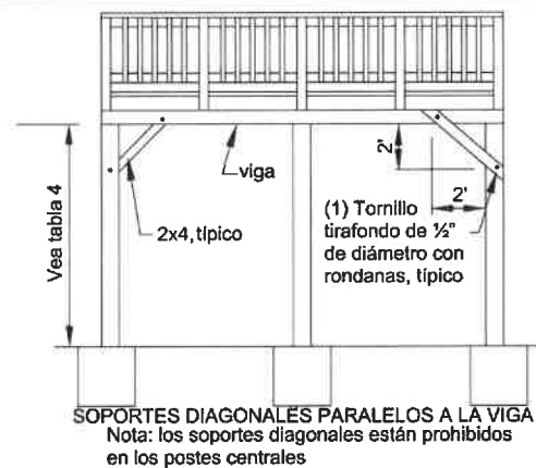
Figura 10. Soportes Diagonales.
