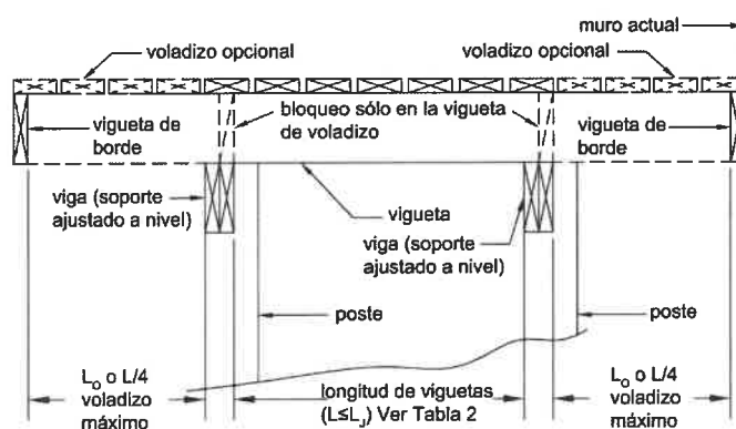
Figura 2. Longitud de Viguetas – Cubiertas sin Largueros.
