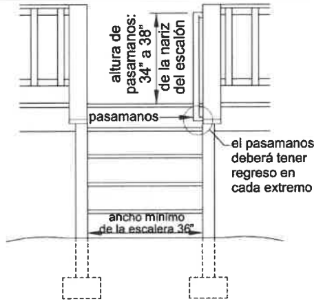
Figura 33. Requerimientos Misceláneos para Escalera.
