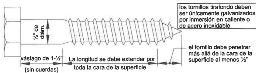
Figura 20. Requerimientos de Tornillos Tirafondo.
