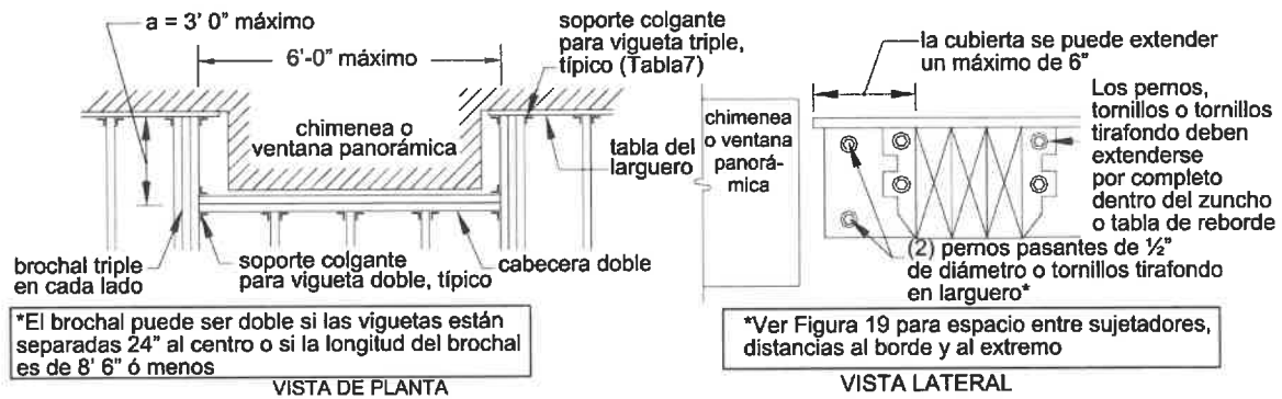
Figura 35. Detalles para Estructuras Alrededor de una Chimenea o de una Ventana Panorámica.
