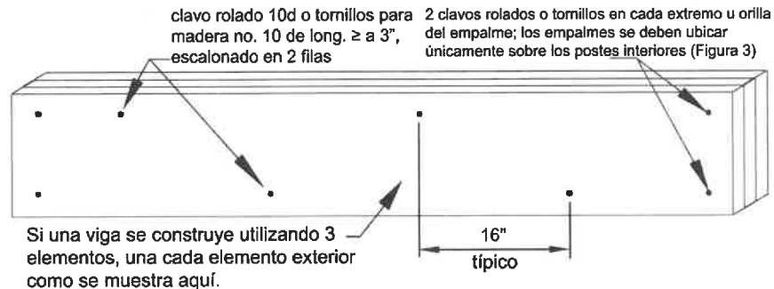
Figura 4. Detalles de Ensamble de Viga.
