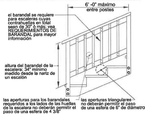
Figura 30. Requerimientos del Barandal.
