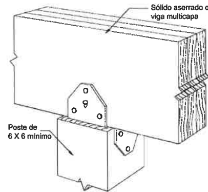
Figura 9. Condición de Unión Prohibida Poste-a-Viga.
