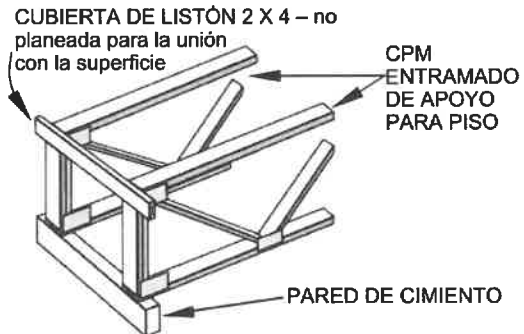
Figura 14. Unión General de la Tabla del Larguero a la Viga del Borde o Remate de la Vigueta.
