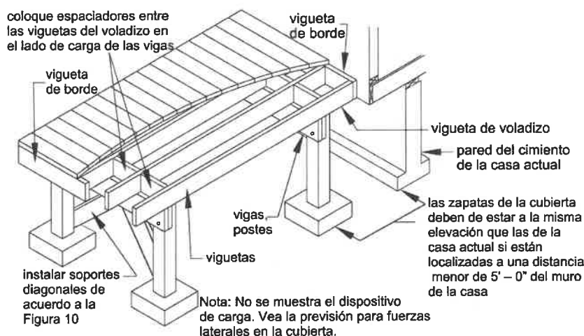
Figura 21. Cubierta sin Largueros – Para Resistir Cargas Verticales.
