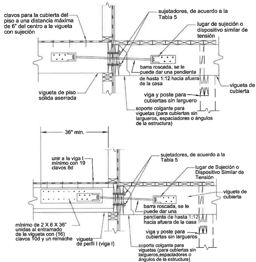
Figura 23. Dispositivo de Carga Lateral con Piso de Viguetas Perpendiculares a las Viguetas de la Cubierta.
