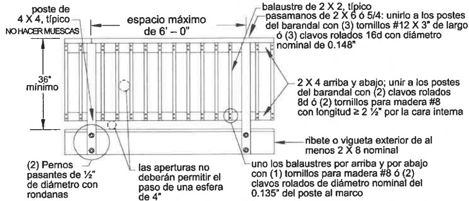
Figura 24. Detalle de Ejemplo de Barandal.
