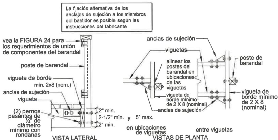
Figura 26. Ejemplo de Poste de Barandal con Vigüeta de Borde.
