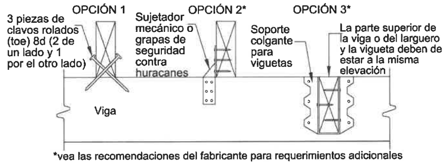
Figura 6. Detalle Vigueta-a-Viga.
