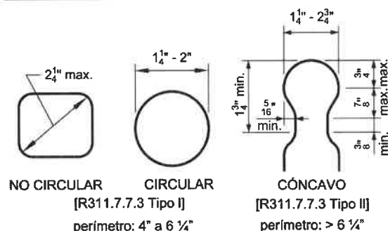
Figura 32B. Tamaño de Asidero de Pasamanos.
