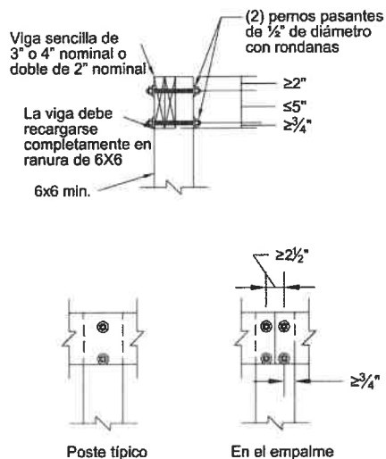
Figura 8A. Requerimientos de unión Poste a Viga.
