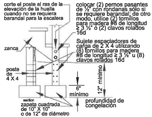
Figura 34. Detalle de Zapatas para Escalera.
