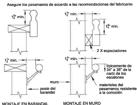
Figura 32A. Ejemplos de Montaje de Pasamanos.
