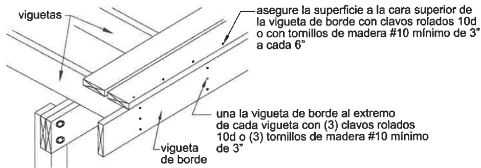
Figura 11. Detalles de Conexión de Vigueta de Borde.
