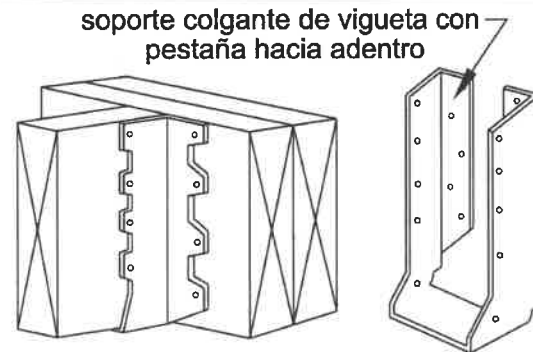
Figura 7. Típico Soporte Colgante de Vigueta.
